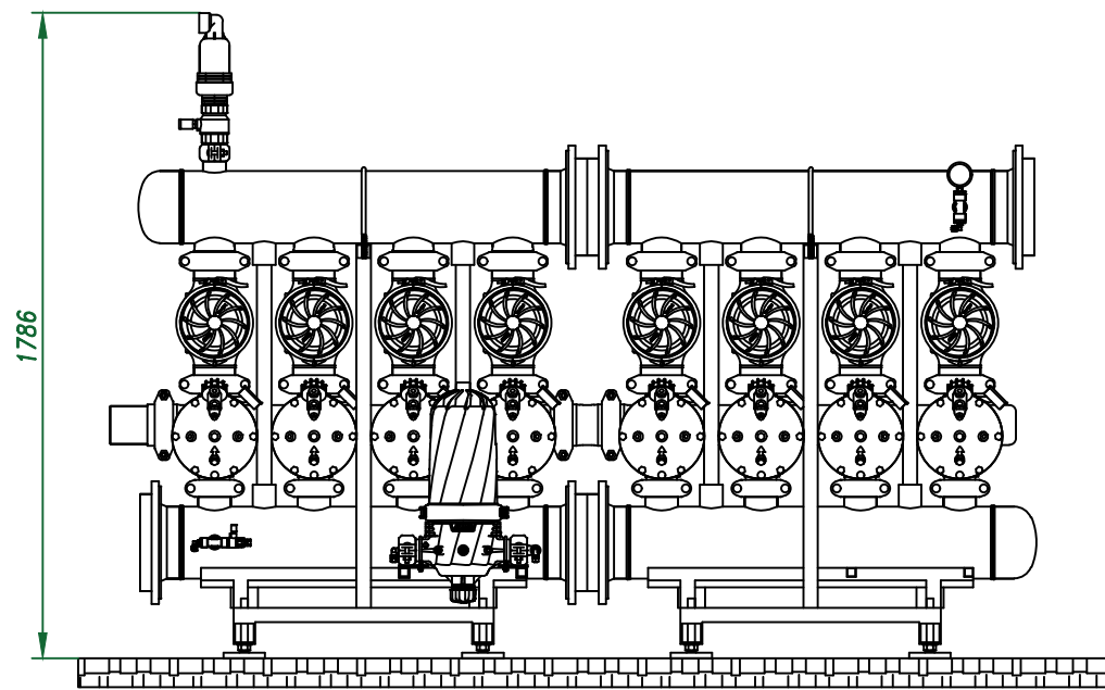
Вид спереди
